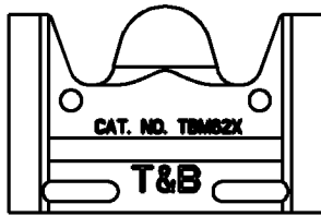
Upper Indenter
